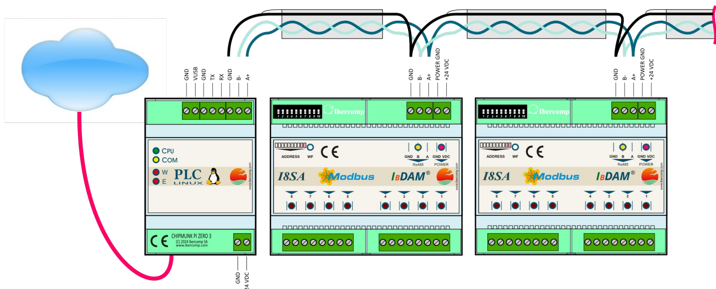
Instalación basada en autómata, PLC o microcotrolador
